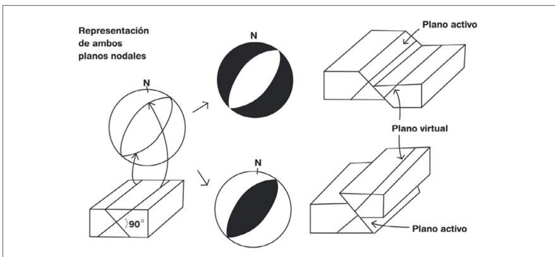
Fig. 27: Correlación entre el cambio de la dirección de desplazamiento sobre el plano de falla y la distribución de primeros impulsos. Obsérvese que la inclinación de los planos nodales en el diagrama no se modifica. Compárese con el gráfico que indica que los planos de fractura compresiva forman un ángulo menor de 45° con el eje de esfuerzo compresivo mayor, mientras que los planos de fractura extensiva forman un ángulo mayor de 45° con el eje extensivo. Como lo que importa es que los ejes de esfuerzos son bisectrices de los planos nodales, en realidad la simplificación no modifica la posición espacial de los mismos.
