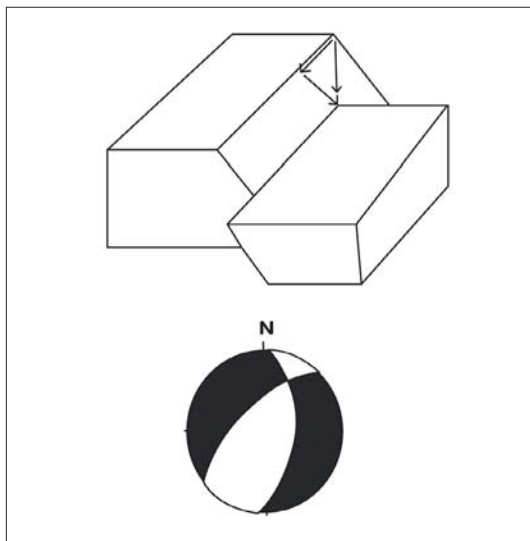
Fig. 20: Falla directa con componente de desplazamiento dextral
