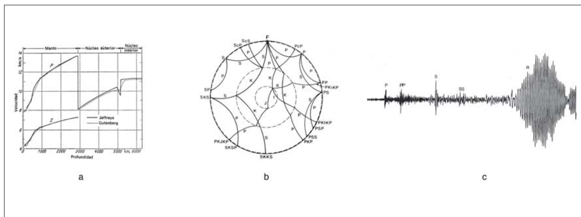
Fig. 2: a) Variación de la velocidad de las ondas sísmicas con la profundidad. b) Debido a la variación sistemática de la velocidad de las ondas sísmicas con la profundidad (como consecuencia de la variación conjunta de la presión, la temperatura, la composición y la densidad de los materiales) éstas se refractan y reflejan, pudiendo recorrer diferentes caminos. Se ha desarrollado una nomenclatura particular para describir dichos caminos. Así las letras P y S se refieren a las ondas longitudinales y transversales que atraviesan el manto y el núcleo. La letra K corresponde al tramo de la trayectoria de una onda P que se localiza en el núcleo externo, mientras que la I representa el tramo que lo hace en el núcleo interno. En el caso de las ondas S , éstas no se propagan en el núcleo externo, por comportarse éste como un líquido, pero sí lo hacen en el núcleo interno, recibiendo este tramo de su trayectoria la denominación J . Con las letras minúsculas c e i se identifican las ondas que se reflejan en la interfase manto núcleo y núcleo interno-externo respectivamente. Es importante que al producirse la reflexión de una onda P sobre la interfase manto-núcleo se generan dos ondas reflejadas: una P y una S . Si no existieran diferencias en la velocidad de transmisión de las ondas sísmicas en el interior de la Tierra todas las trayectorias serían líneas rectas.
