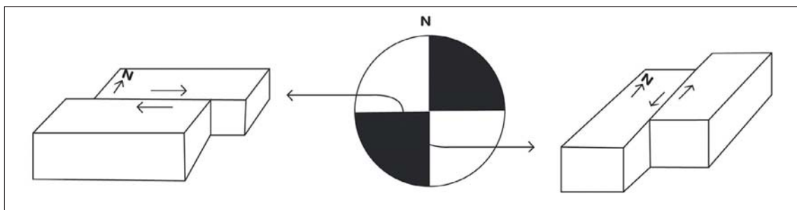
Fig. 22: La clasificación de la falla transcurrente en dextral o sinistral es función del plano que haya sido activo.
