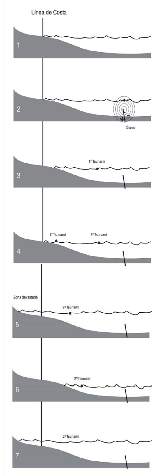
Fig. 11: Esquema que ilustra la generación, propagación y llegada a la costa de una onda Tsunami.
