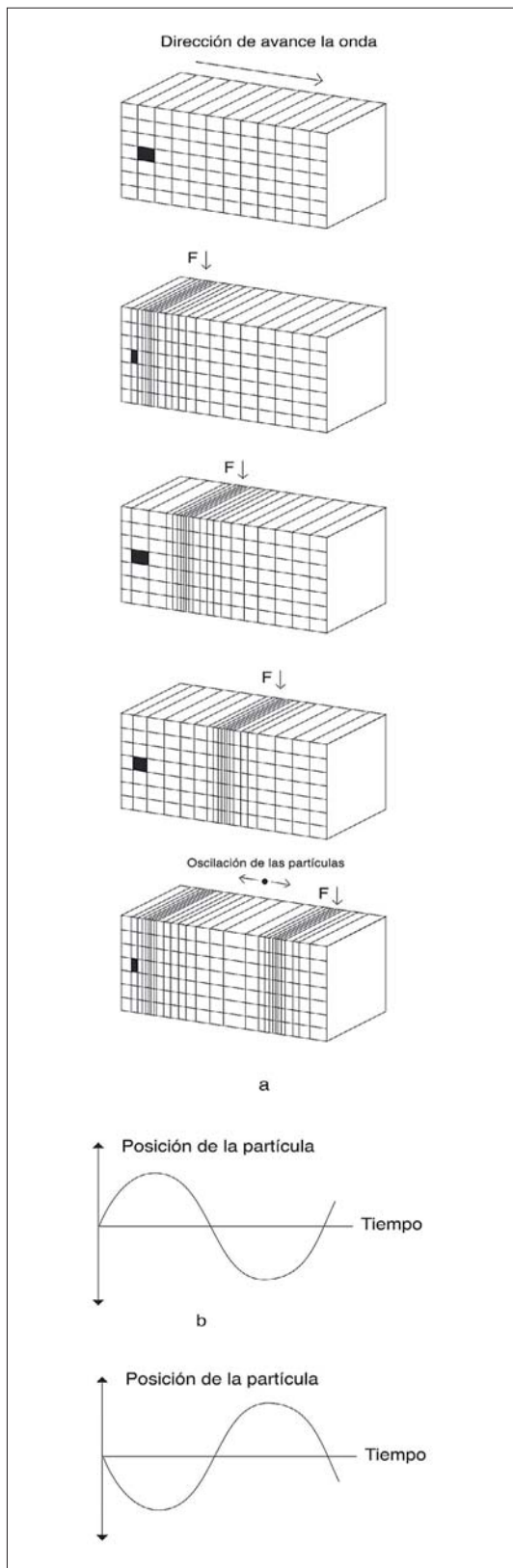
Fig. 4: a) Desplazamiento de una partícula hacia delante y atrás como consecuencia de haber sido alcanzada por una onda de presión. b) Primer arribo compresivo. c) Primer arribo tractivo. En b) y c) el eje vertical representa distancias por delante y por detrás del punto de reposo.
