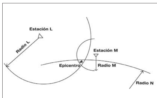
Fig. 9: Determinación de la posición del epicentro por el punto de intersección de los círculos determinados para tres estaciones sismológicas.
