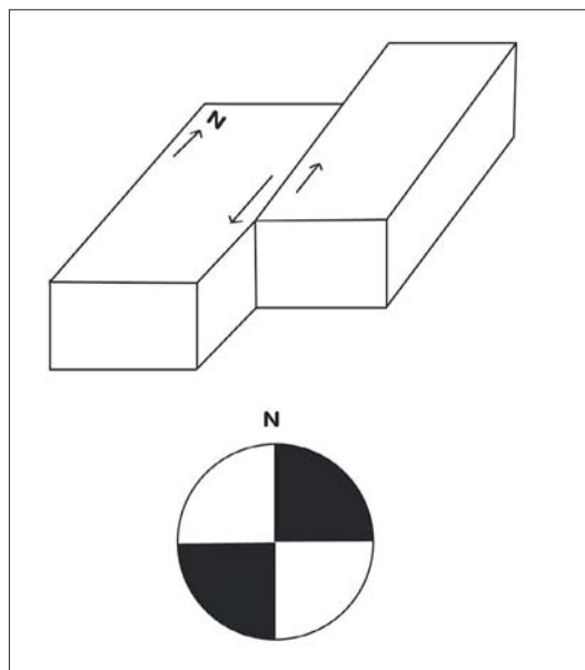
Fig. 19: Falla transcurrente y diagrama del mecanismo focal correspondiente, corte horizontal y corte vertical perpendicular al rumbo de la estructura.
